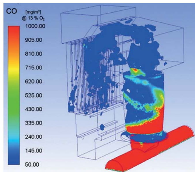
Abbildung 10: Schneckenbrenner für aschereiche Biomassebrennstoffe in Anwendungen von 100–300 kW (Barroso et al. 2019b). Links: Das Prinzip des Schneckenbrenners ermöglicht eine kontinuierliche Entfernung der Asche aus der Verbrennungszone, um das Schmelzen und die Ablagerung von Asche zu vermeiden, was die Verwendung von aschereichen Brennstoffen in konventionellen Kleinkesseln unmöglich macht. Rechts: CO-Konzentration als Beispiel für die Ergebnisse der numerischen Fluidodynamikmodellierung (Barroso et al. 2019c). Die Modellierung der Strömungsdynamik und Experimente werden zur Optimierung der Lufteinblasung und der Verbrennungsgeometrie eingesetzt, um eine Verbrennung mit minimalem Luftüberschuss und folglich höherem Wirkungsgrad zu ermöglichen und die Schadstoffemissionen, insbesondere unverbrannte kohlenstoffhaltige Verbindungen und Stickoxide ( \text{NO}_x ), zu verringern.
