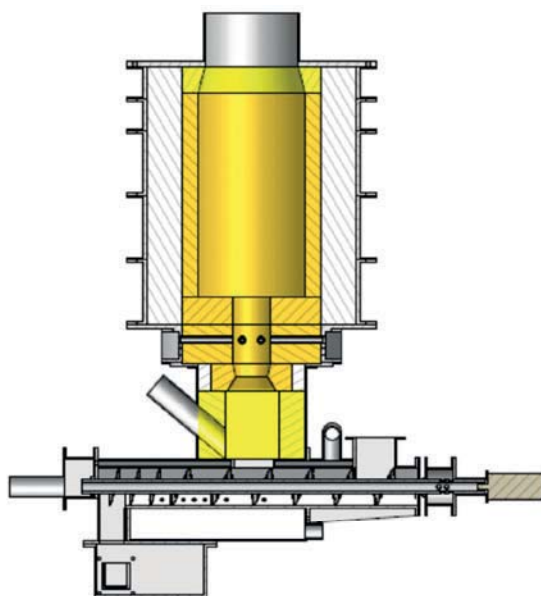
Abbildung 10: Schneckenbrenner für aschereiche Biomassebrennstoffe in Anwendungen von 100–300 kW (Barroso et al. 2019b). Links: Das Prinzip des Schneckenbrenners ermöglicht eine kontinuierliche Entfernung der Asche aus der Verbrennungszone, um das Schmelzen und die Ablagerung von Asche zu vermeiden, was die Verwendung von aschereichen Brennstoffen in konventionellen Kleinkesseln unmöglich macht. Rechts: CO-Konzentration als Beispiel für die Ergebnisse der numerischen Fluidodynamikmodellierung (Barroso et al. 2019c). Die Modellierung der Strömungsdynamik und Experimente werden zur Optimierung der Lufteinblasung und der Verbrennungsgeometrie eingesetzt, um eine Verbrennung mit minimalem Luftüberschuss und folglich höherem Wirkungsgrad zu ermöglichen und die Schadstoffemissionen, insbesondere unverbrannte kohlenstoffhaltige Verbindungen und Stickoxide ( \text{NO}_x ), zu verringern.
